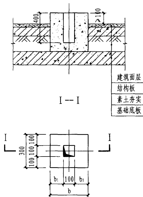
A. 安装在有基础底板地面上的基础图
