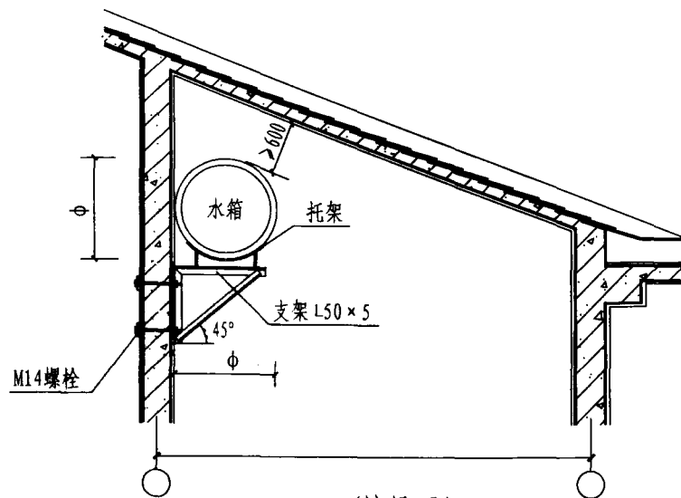
1-1(坡屋面)
