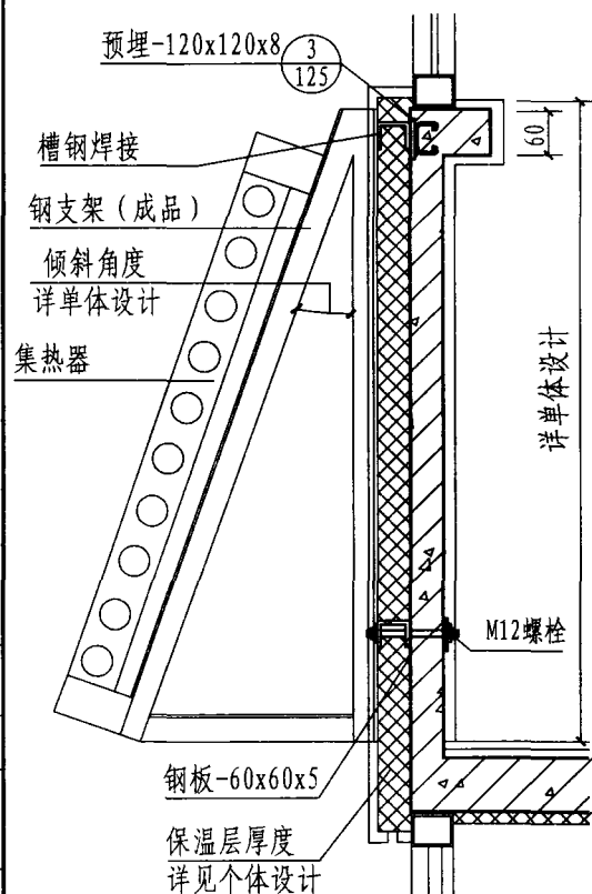
① 倾斜式 (有保温)
