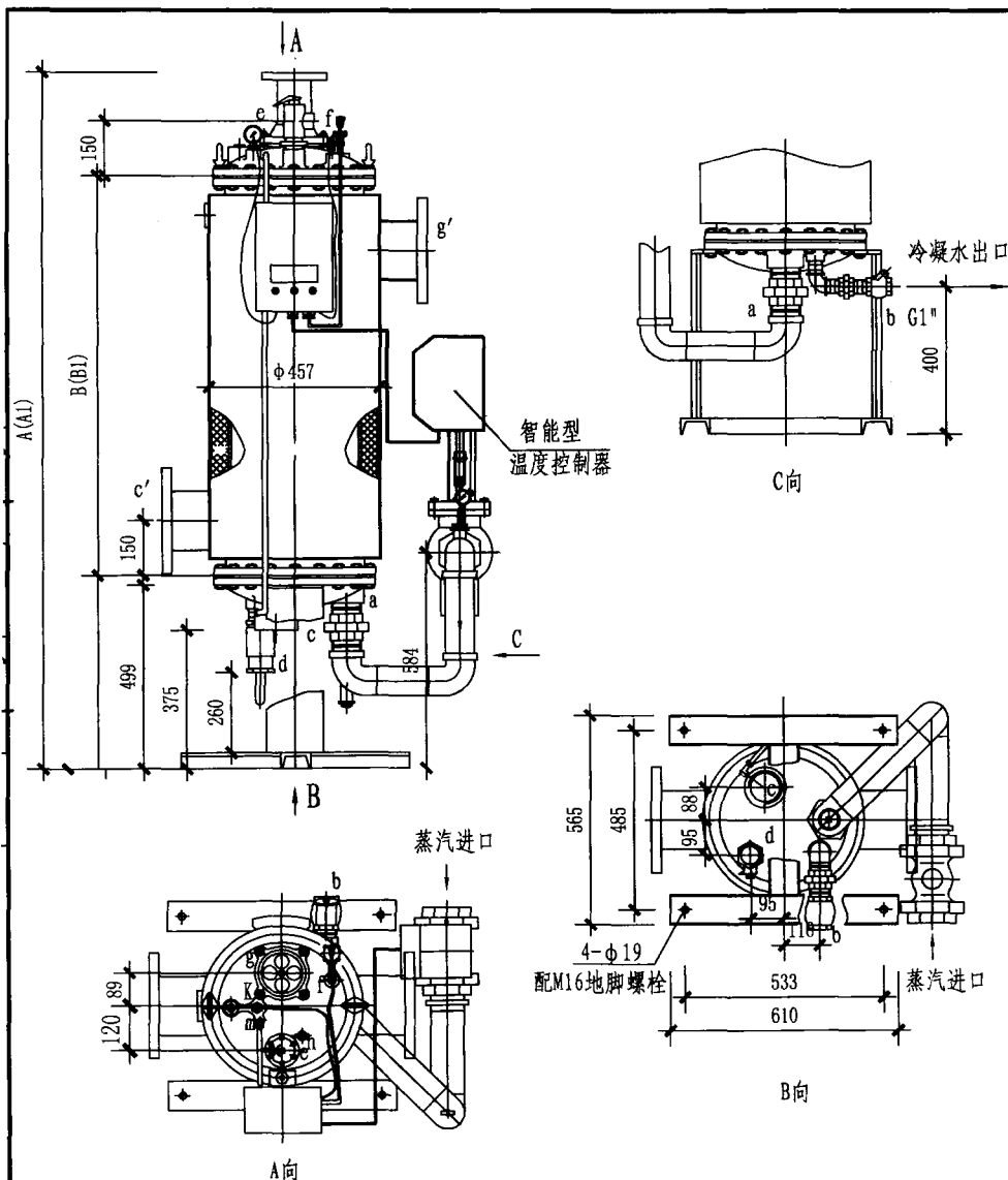
管口表
