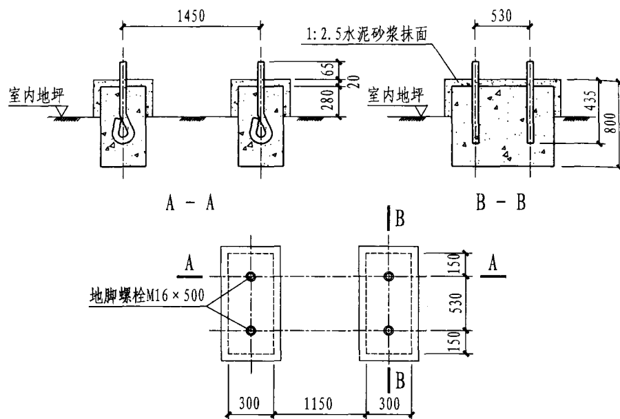
机组基础
