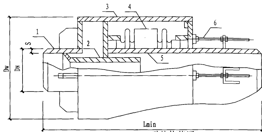
YZ型结构简图
