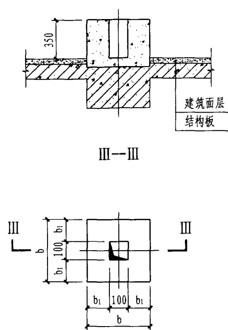
C. 安装在楼板上的基础图
