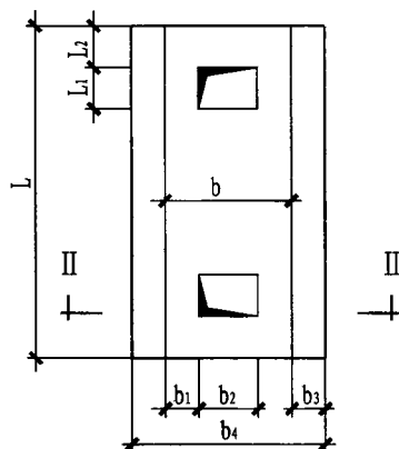
安装在无基础底板地面上的基础图
