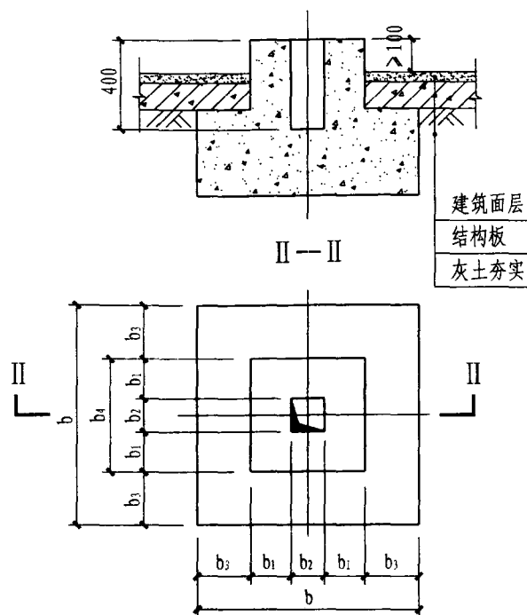
B. 安装在无基础底板地面上的基础图
