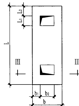
安装在楼板上的基础图
