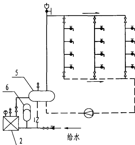
锅炉及冷、热水箱放于屋顶供热水系统
