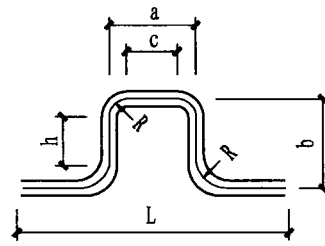
II型
