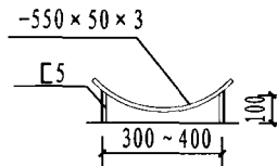
水箱托架
