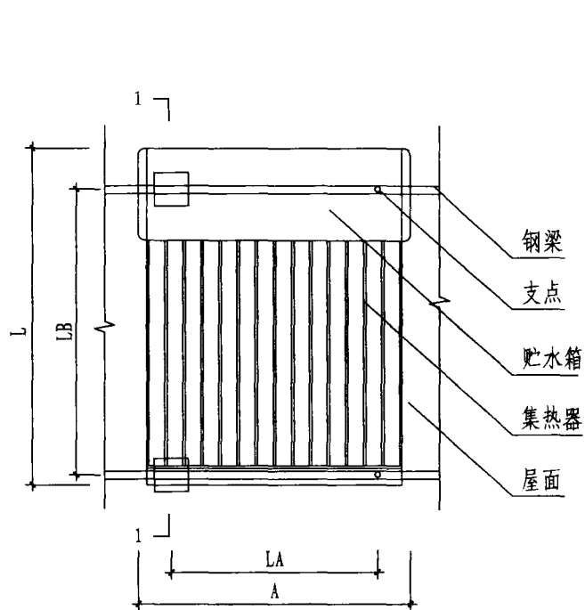
① 平面图
