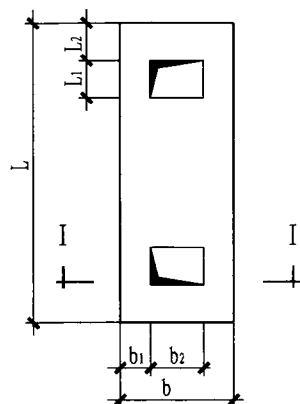
安装在有基础底板地面上的基础图
