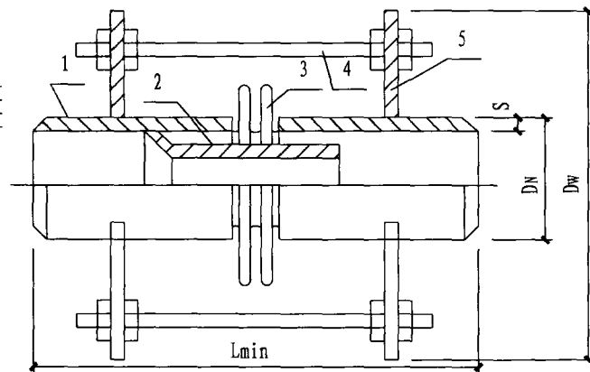
RWZ型结构图
