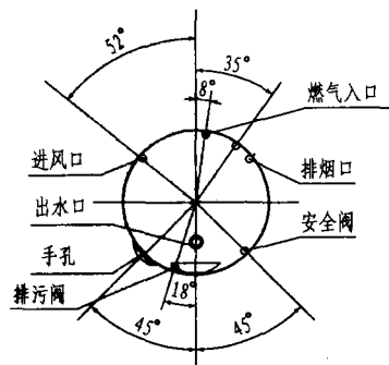
BTH-338系列外形及安装
