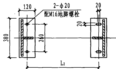
卧式水加热器外形
