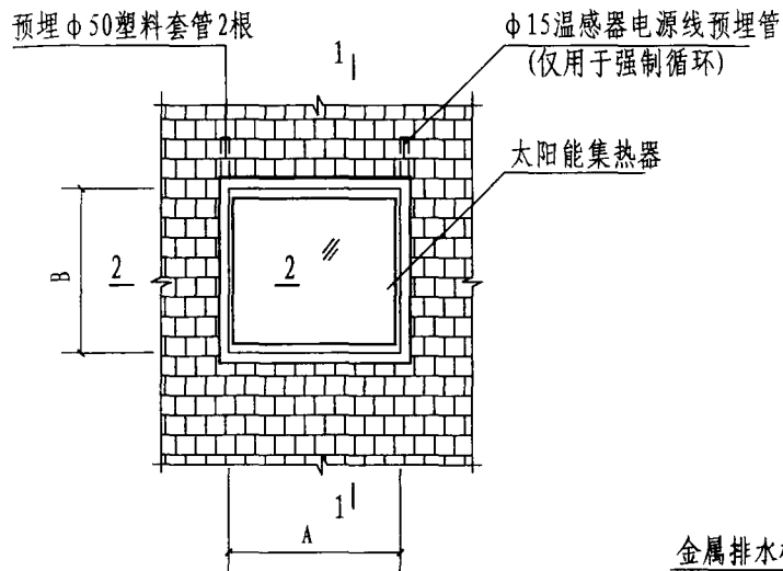
1 平面图
