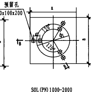
SQL (PN) 立式储水罐、水箱外形及基础尺寸图
