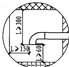
风帽排气口安全间距示意图
