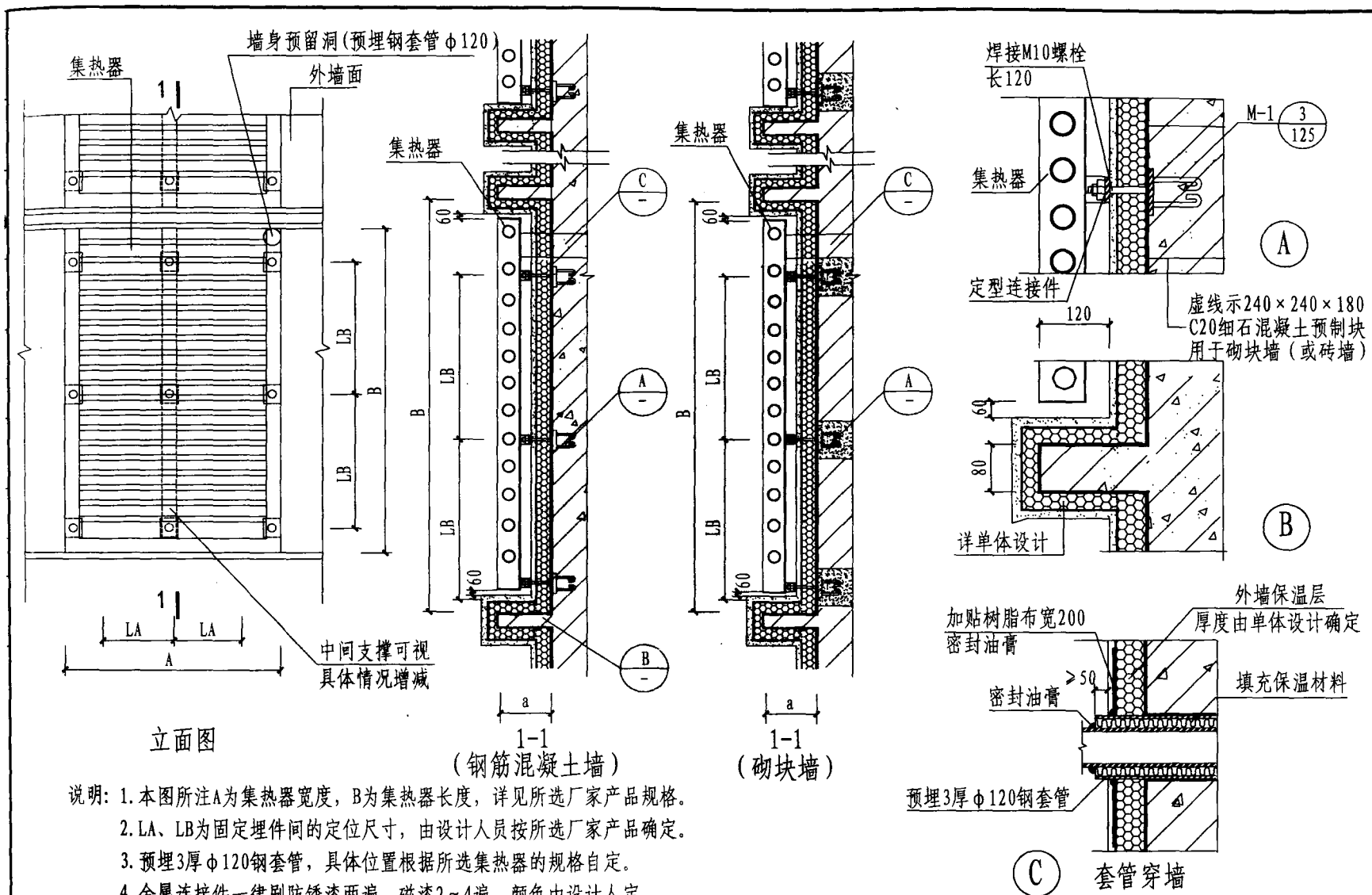
混凝土墙、砌块墙面集热器安装详图
